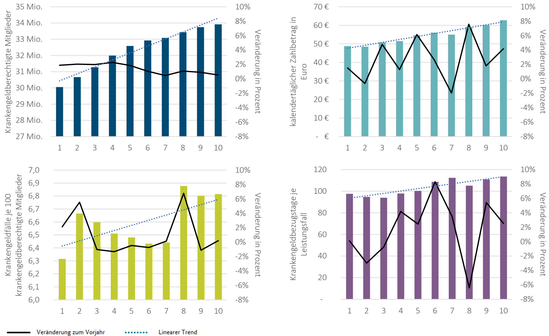
Abbildung 6.9.1.2: Kostentreiberanalyse Krankengeld
