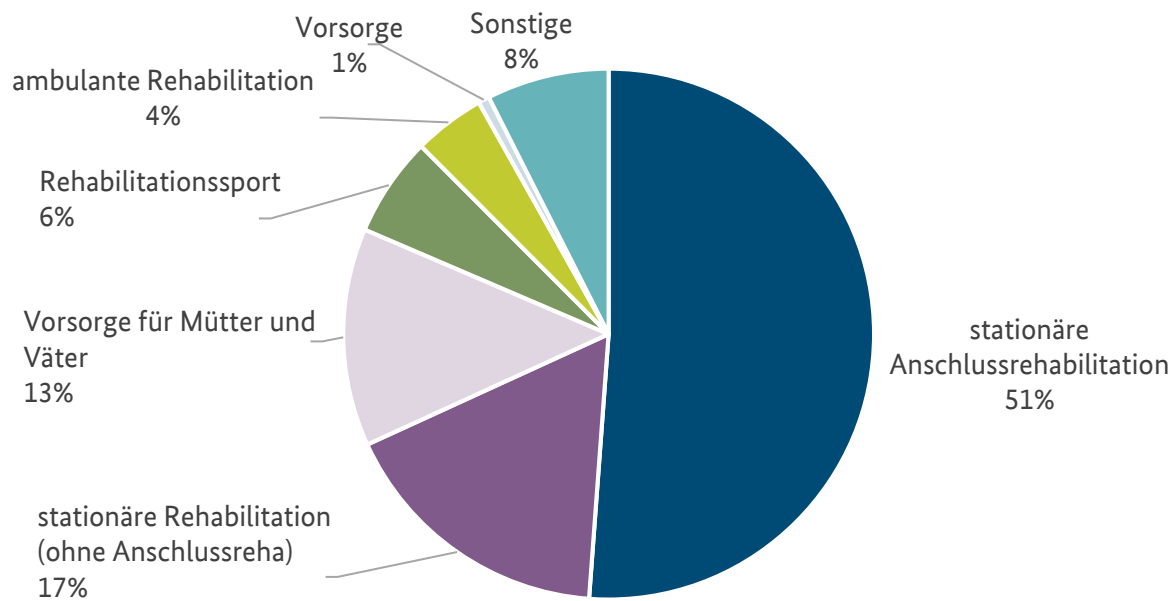
Abbildung 6.10.1.4: Verteilung der Ausgaben im Leistungsbereich „Vorsorge und Rehabilitation“ für 2024
