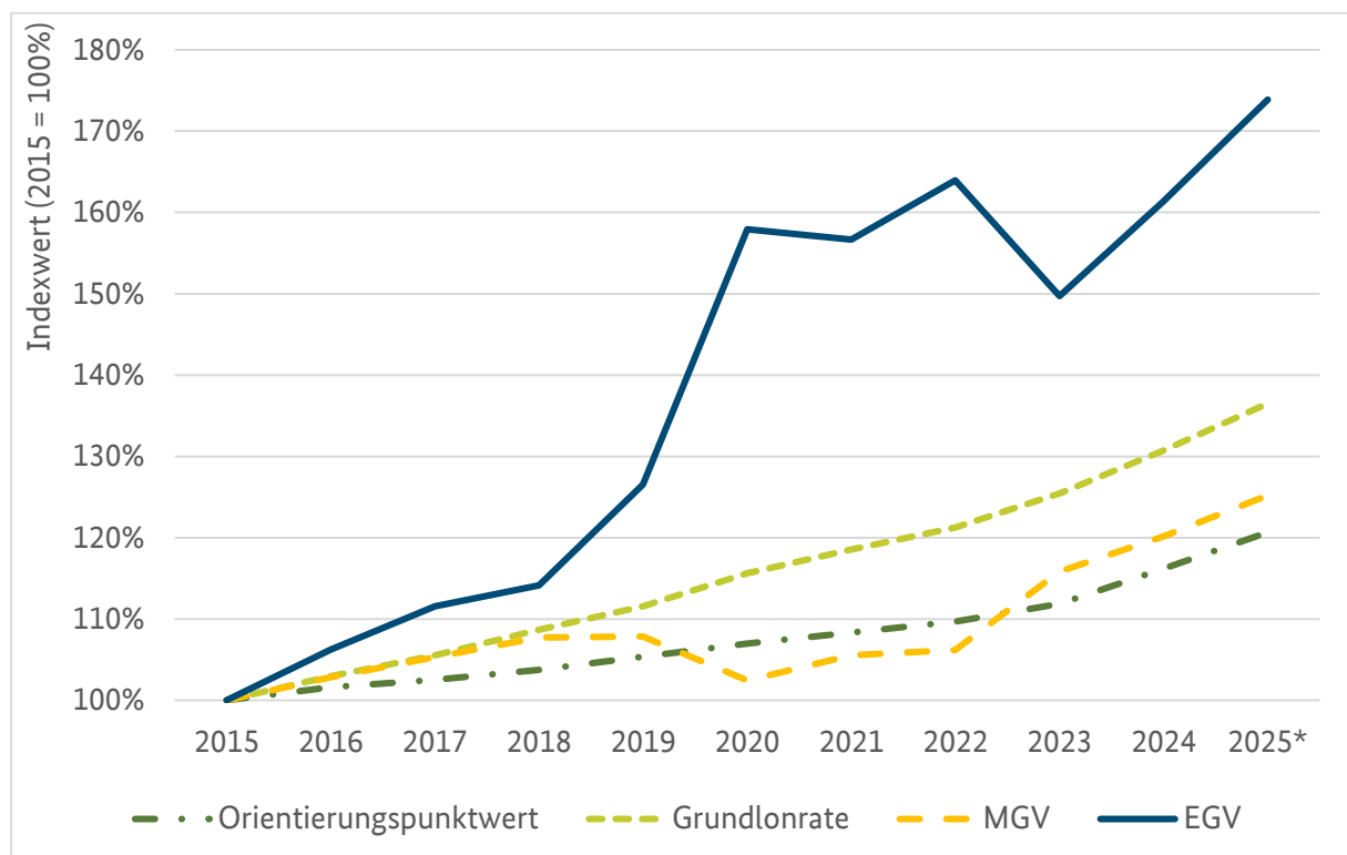
Abbildung 6.3.8.1 Indexierte Ausgabenentwicklung in der vertragsärztlichen Versorgung nach EGV und MGW von 2015 bis 2025 12
