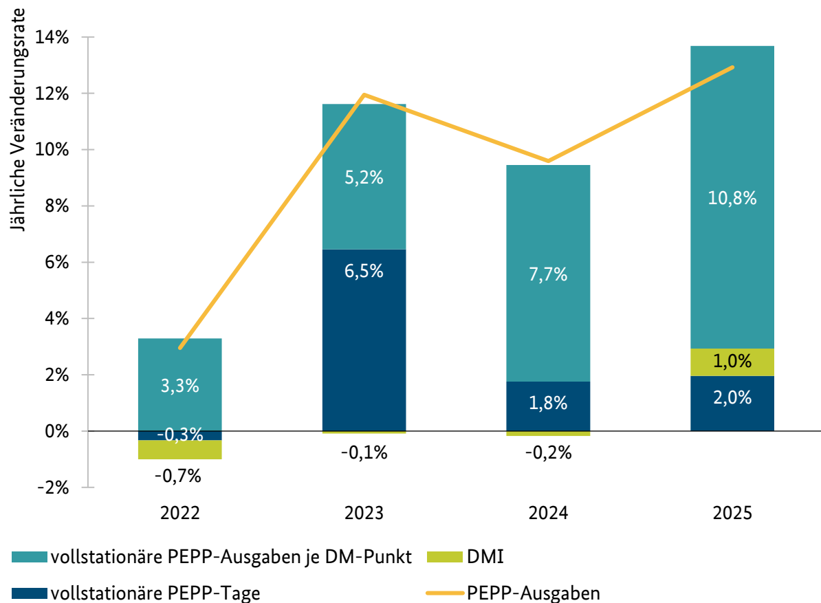
Abbildung 6.6.1.3: Komponentenzerlegung im vollstationären PEPP-Bereich (2021-2025)
