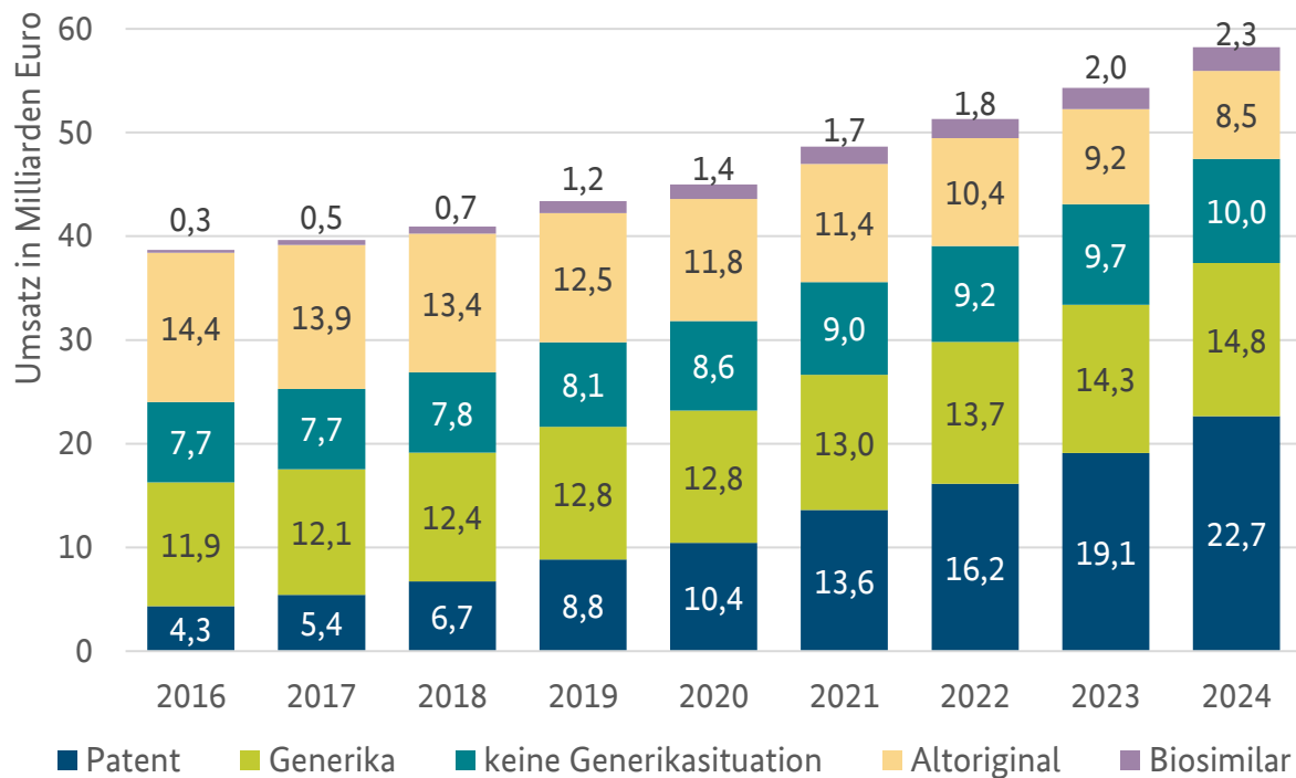
Abbildung 6.7.1.2: GKV-Arzneimittelumsatz nach Marktsegmenten
