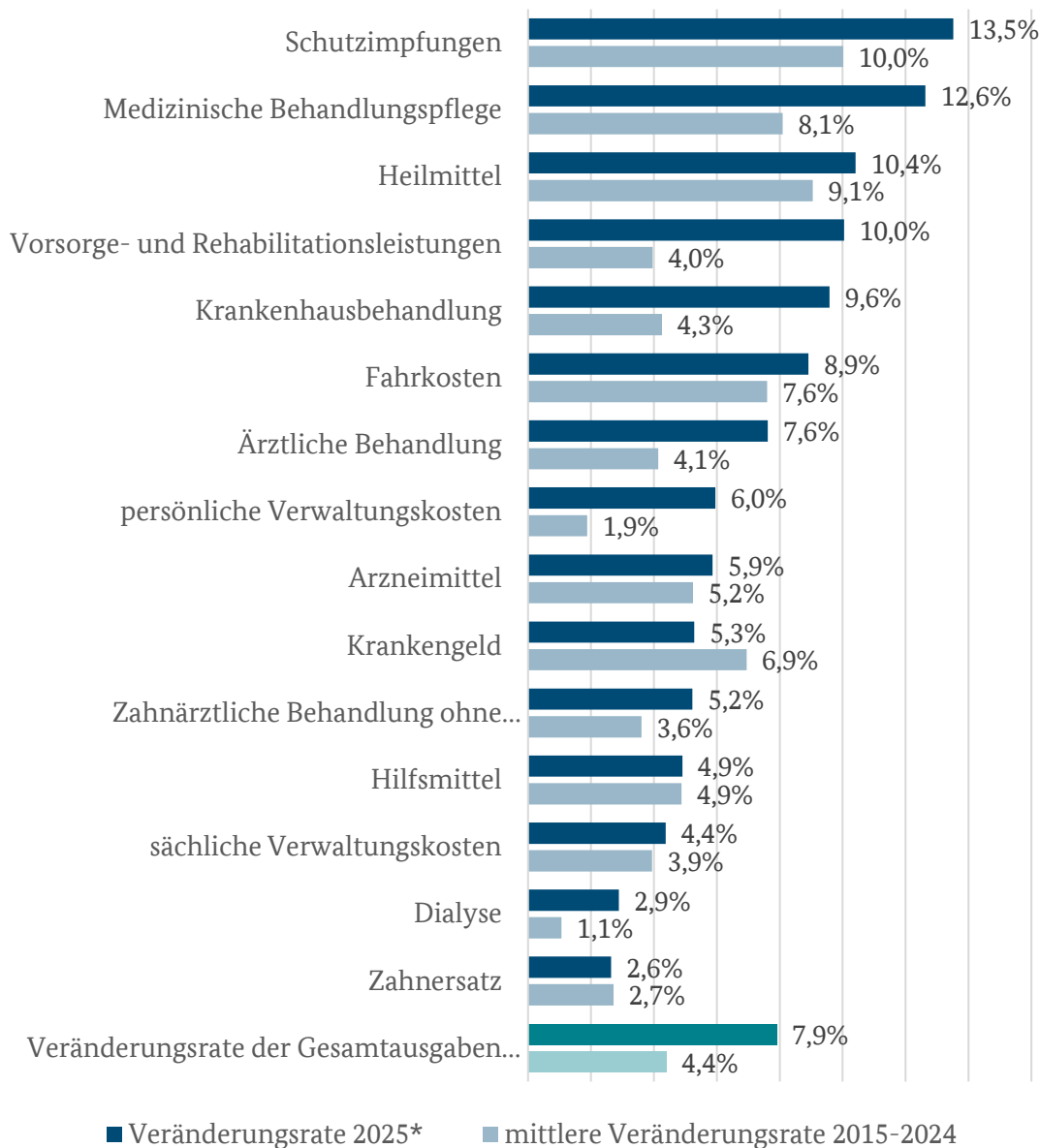
Abbildung 4.1.1.2: Entwicklung der Veränderungsraten der GKV-Ausgaben nach Leistungsbereichen
