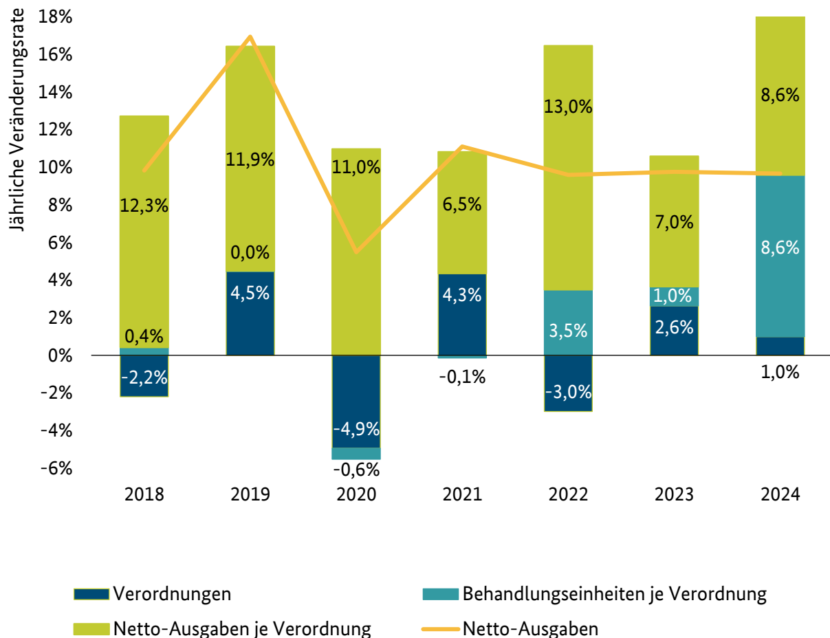
Abbildung 6.5.1.3: Komponentenerzerlegung im Heilmittelbereich (2017-2024)
