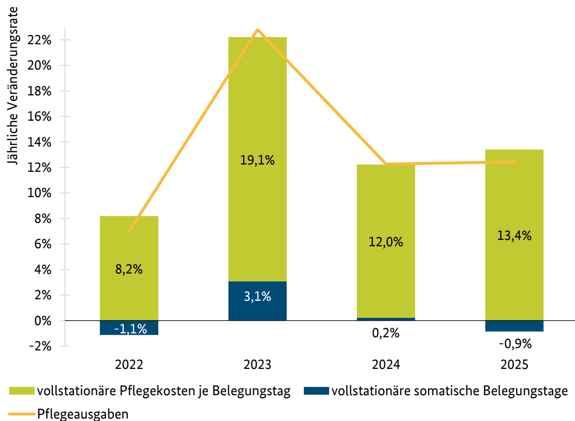
Abbildung 6.6.1.4: Komponentenzerlegung im vollstationären, somatischen Pflegebereich (2021-2025)
