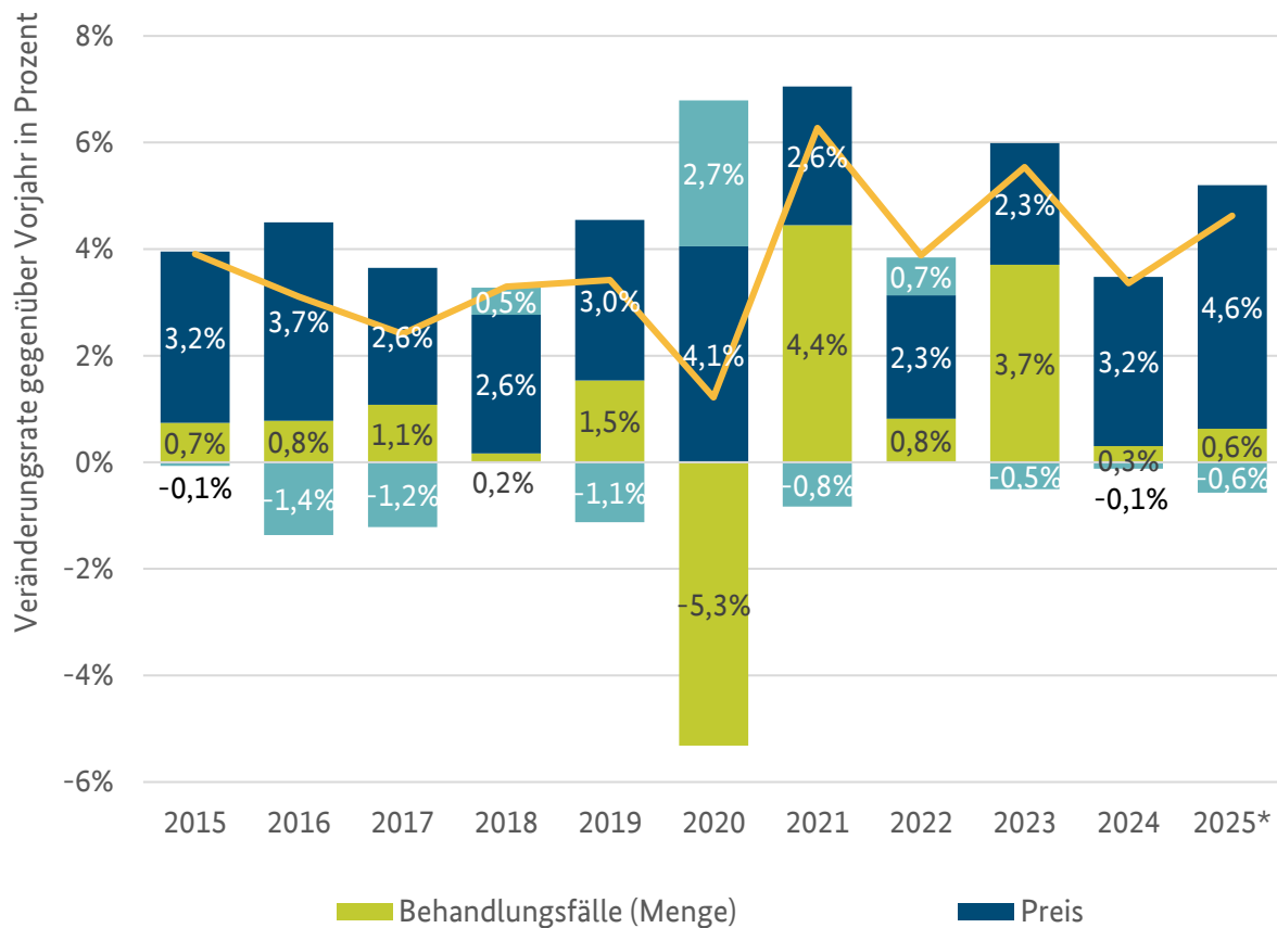
Abbildung 6.4.1.2: Veränderungsraten der Preis-, Mengen und Strukturkomponente für Zahnärzte ohne Zahnersatz von 2015 bis 2025
